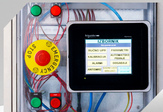
Alta Pro 42: upravljački zaslon
