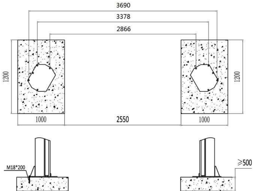
ВАРИАНТ 2 – фундамент на отделни стъпки
