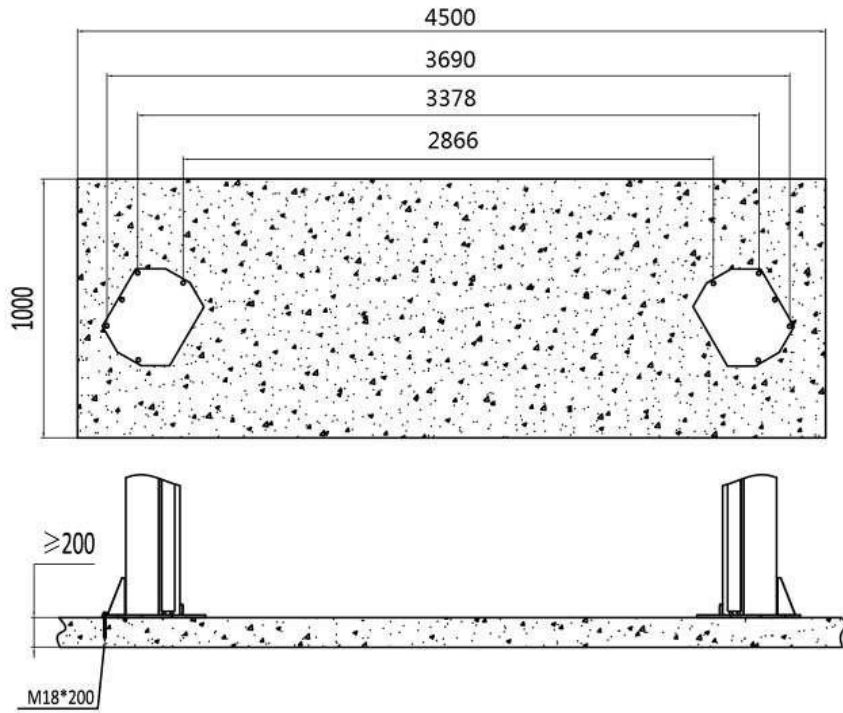
ВЕРСИЯ 1 – фундамент на цяла плоча
