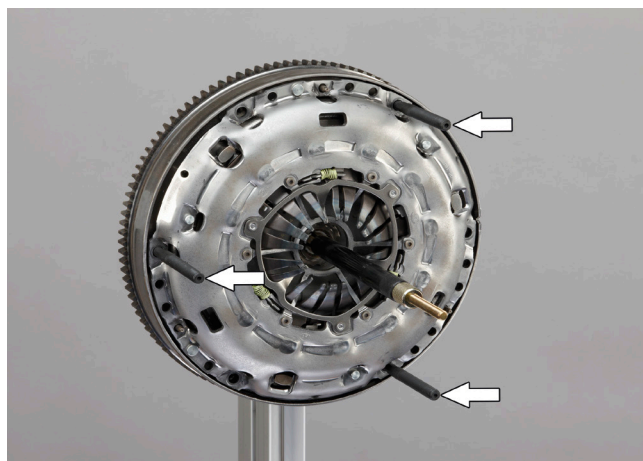
2. ábra: Tőcsavar az orsó tartójának a felfogására
