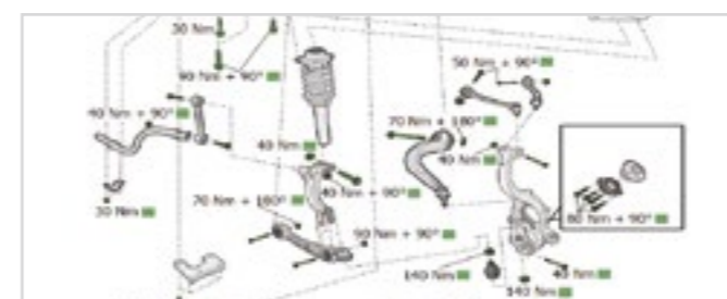
Tehnički nacrti sa integriranim zakretnim momentima
