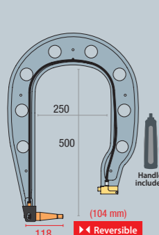
G4 8 bar/550 daN 022799
