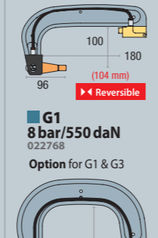
G1 8 bar/550 daN 022768
