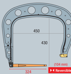
G8 8 bar/550 daN 022836
