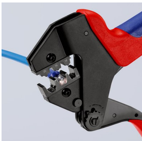
97 43 200 z matrycą do zagniatania 97 49 06 do izolowanych końcówek kablowych, końcówek nasuwanych i łączników kablowych
