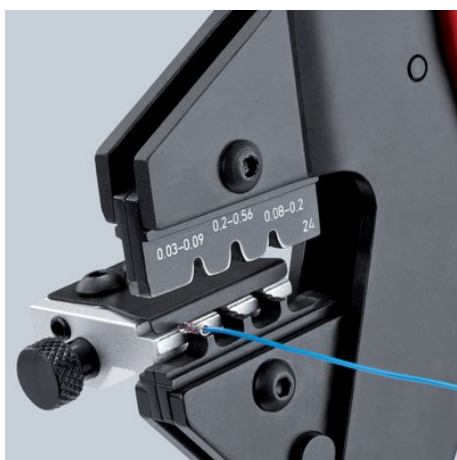
Szczypce do zagniatania typu Crimp System 97 43 200 z matrycą 97 49 24 do złącz wtykowych D-Sub
