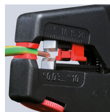
12 40 200: Απογύμνωση ακριβείας αποκλείει οποιονδήποτε τραυματισμό του αγωγού
