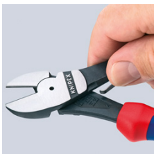
74 12: Το ελατήριο ανοίγματος ενεργοποιείται απλά με την πίεση του αντίχειρα
