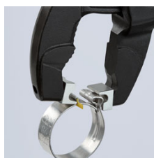
Zatvaranje obujmice za crijevo bez graničnika
