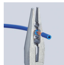
skidanje izolacije
