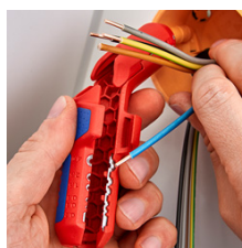
Απογύμνωση ξεχωριστών αγωγών
