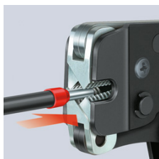
Čeono uvođenje završnih čahura za žile npr. u rasklopnim ormarima
