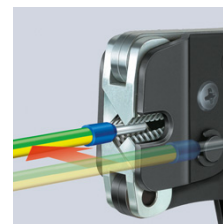
97 53 08: uvođenje završnih čahura za žile paralelno sa strane do 2,5 mm 2 , npr. u skučenim prostorima
