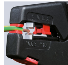
12 40 200: Απογύμνωση ακριβείας αποκλείει τραυματισμό του αγωγού
