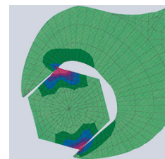
Uobičajeni ključ za vijke: Pritiskanje rubova dovodi do oštećenja
