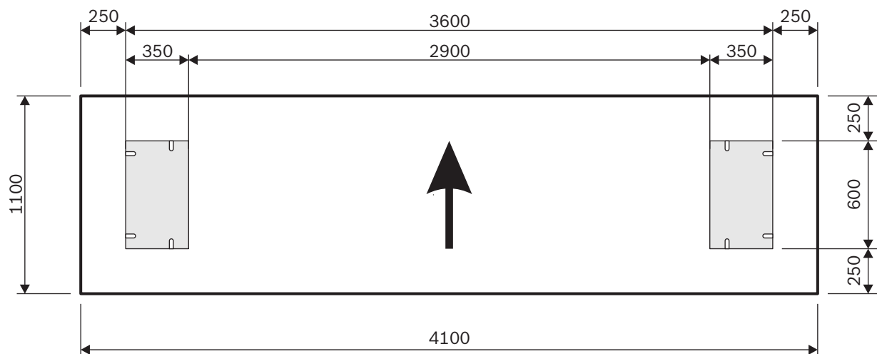
Rys. 31: Plan fundamentu 1 (wymiary w mm; strzałka = kierunek ruchu) Grubość betonu: min. 230 mm.
