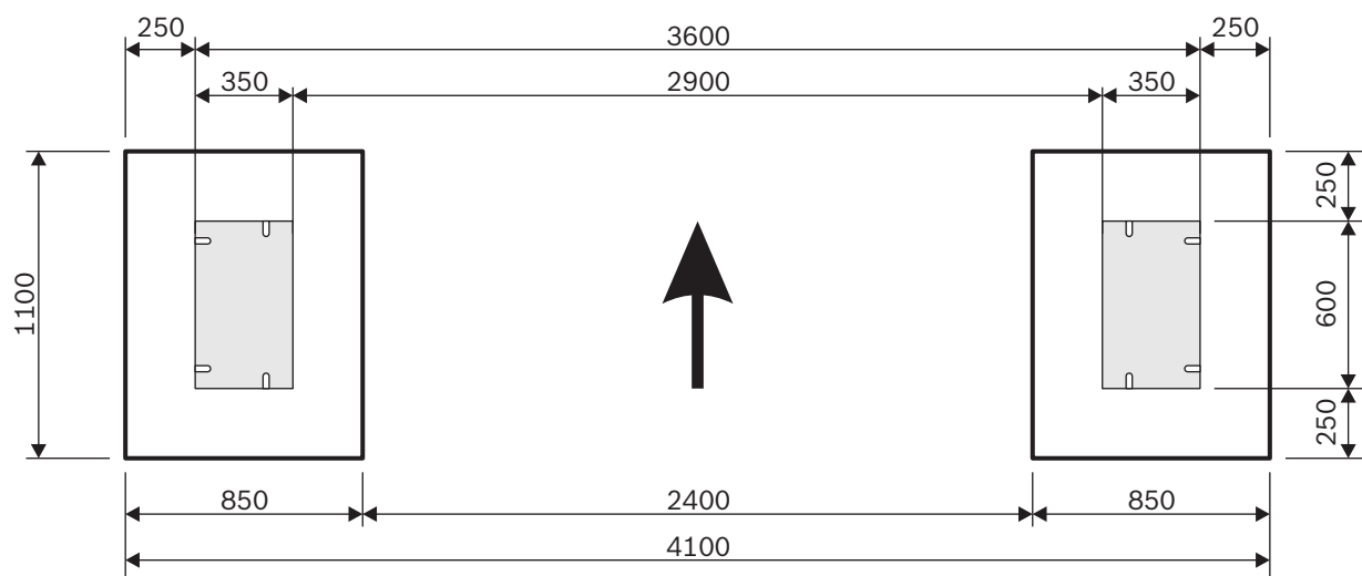
Rys. 32: Plan fundamentu 2 (wymiary w mm; strzałka = kierunek ruchu) Grubość betonu: min. 500 mm.
